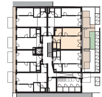
1.OG STRASSENTRAKT
