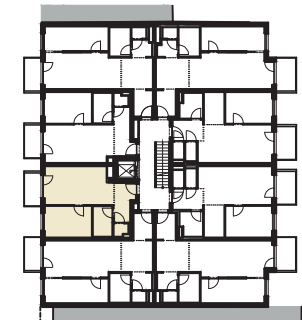
3.OG STRASSENTRAKT
