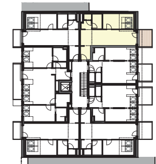
1.DG STRASSENTRAKT
