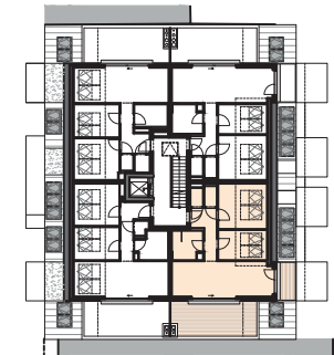
2.DG STRASSENTRAKT
