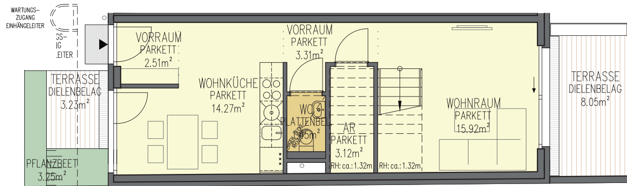
GRUNDRISS 1.OG
