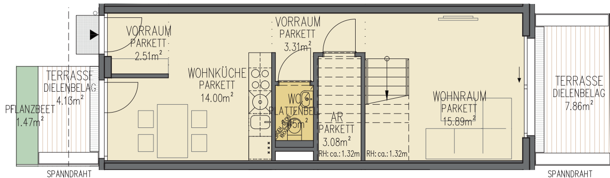
GRUNDRISS 1.OG
