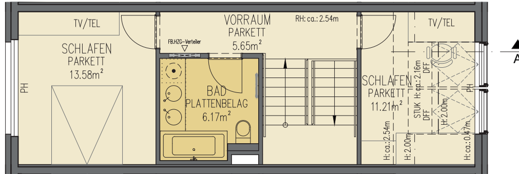
GRUNDRISS 1.DG
