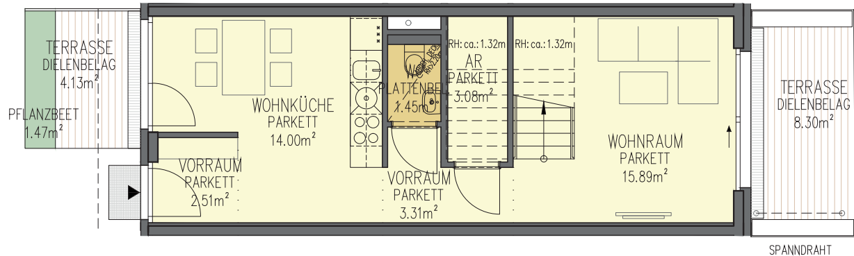
GRUNDRISS 1.OG
