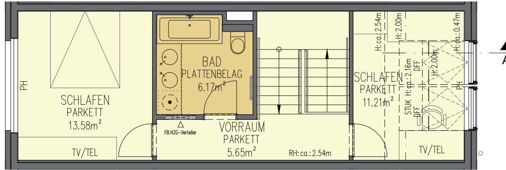
GRUNDRISS 1.DG
