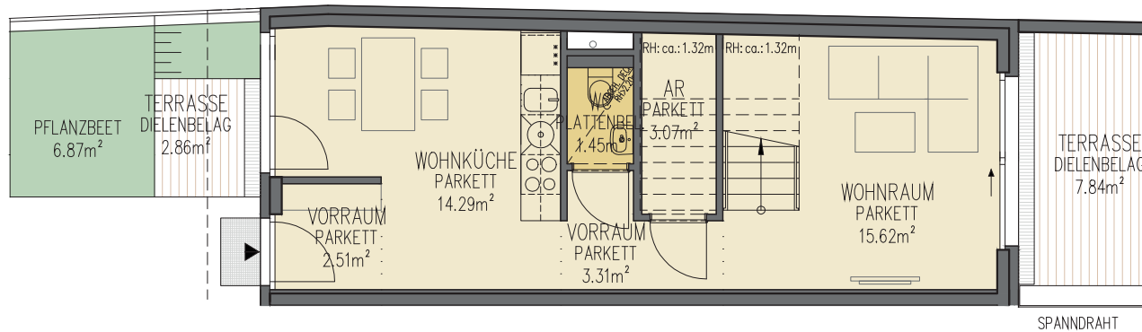
GRUNDRISS 1.OG
