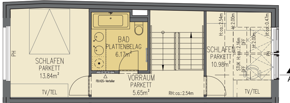
GRUNDRISS 1.DG
